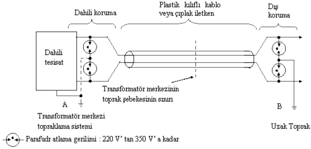
Şekil-Z.1 Koruma için prensip şeması
