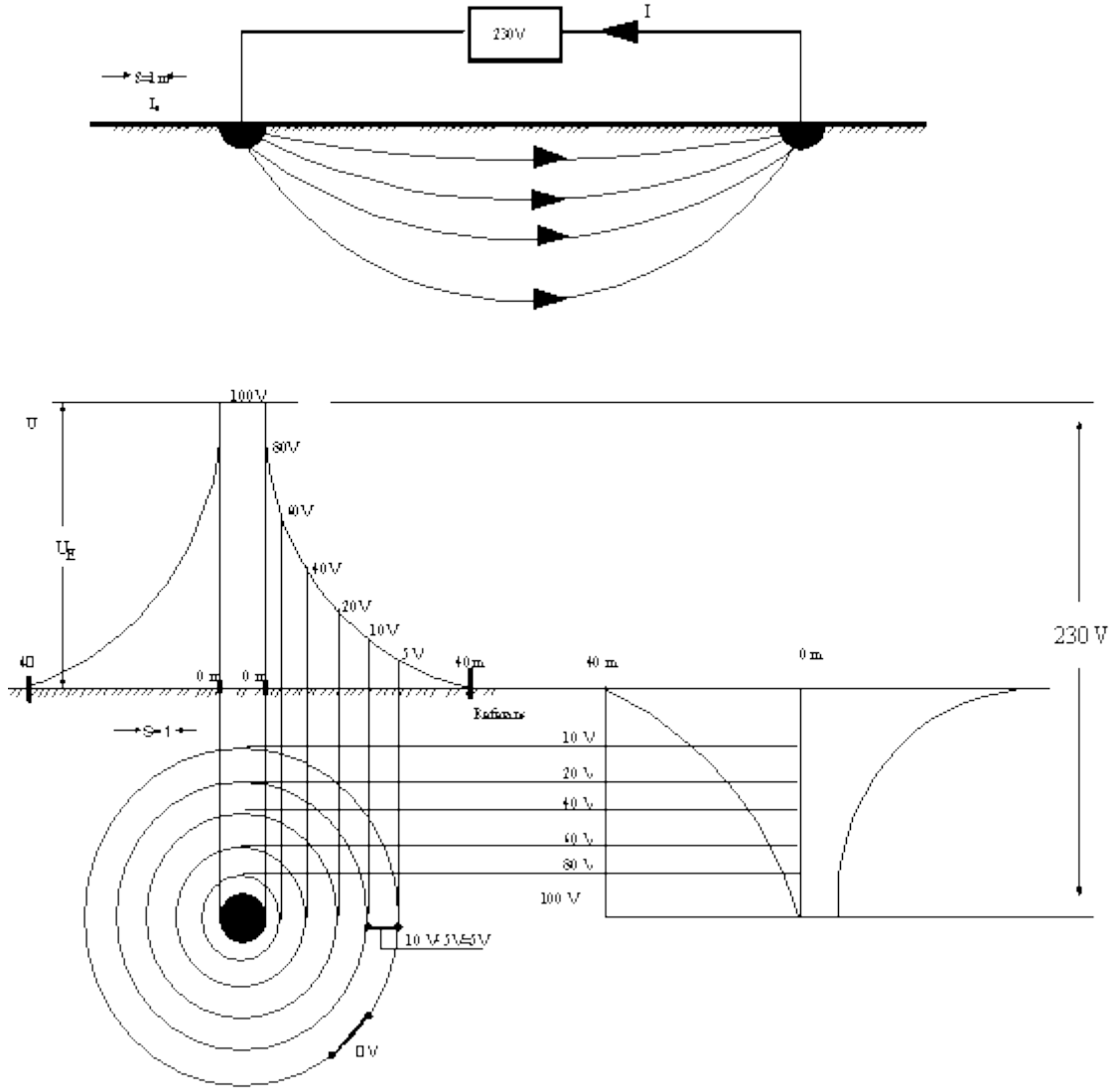
Şekil-T.4 Bir topraklayıcıda yayılma direncinin uzaklıkla değişim
