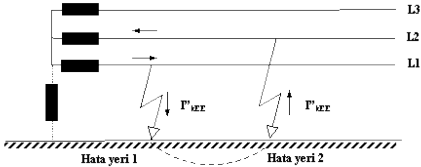
Şekil-4d Toprak teması kompanze edilmiş ve geçici olarak yıldız noktası değeri düşük bir empedans üzerinden topraklanmış bir şebekede toprak hata akımı
