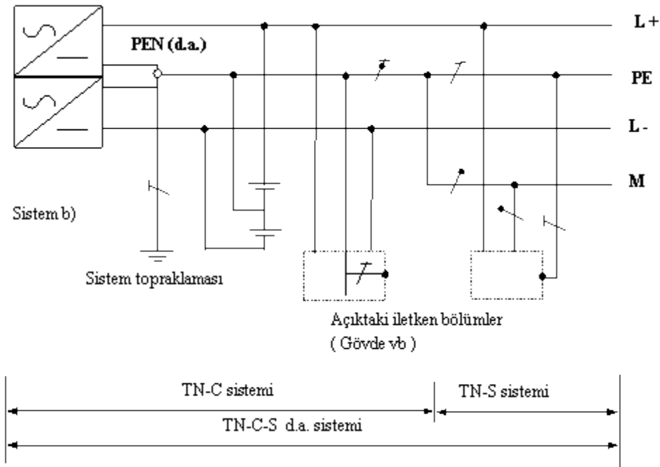
Şekil-5h TN-C-S Doğru akım sistemi
