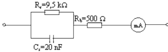
Şekil-11 Küçük yüzeyli temaslarda 100 Hz'in üstündeki periyodik akımların ölçülmesi için bağlantı devresi
