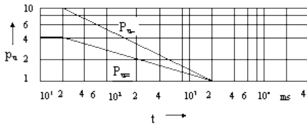
Şekil-Y.8 Etki süresine t bağlı olarak kısa süre katsayıları p_{U\sim} ve p_{U=} 'nin değişimi
