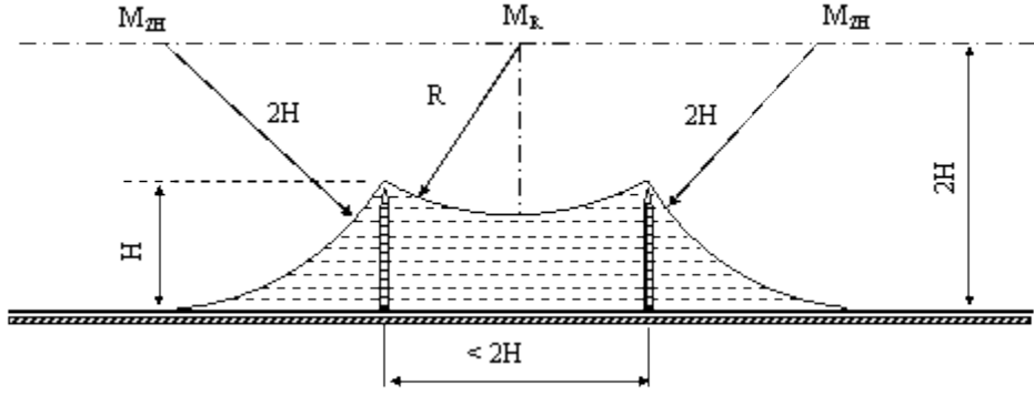
Şekil-H.2 İki koruma teli
