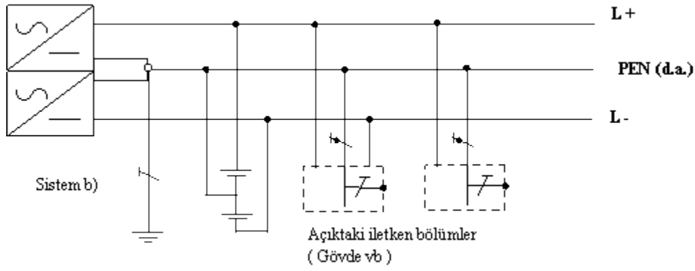
Şekil-5g TN-C Doğru akım sistemi
